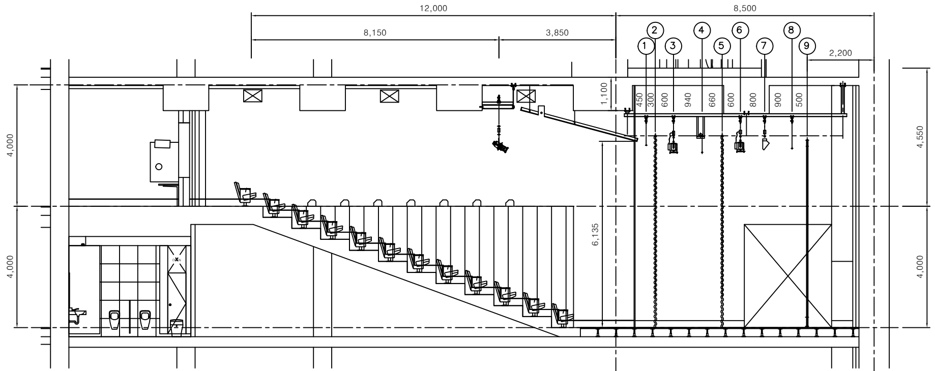
A-C 001 시민이용 소극장 무대기계장치 단면 배치도 축척 : 1/100 (A3)
