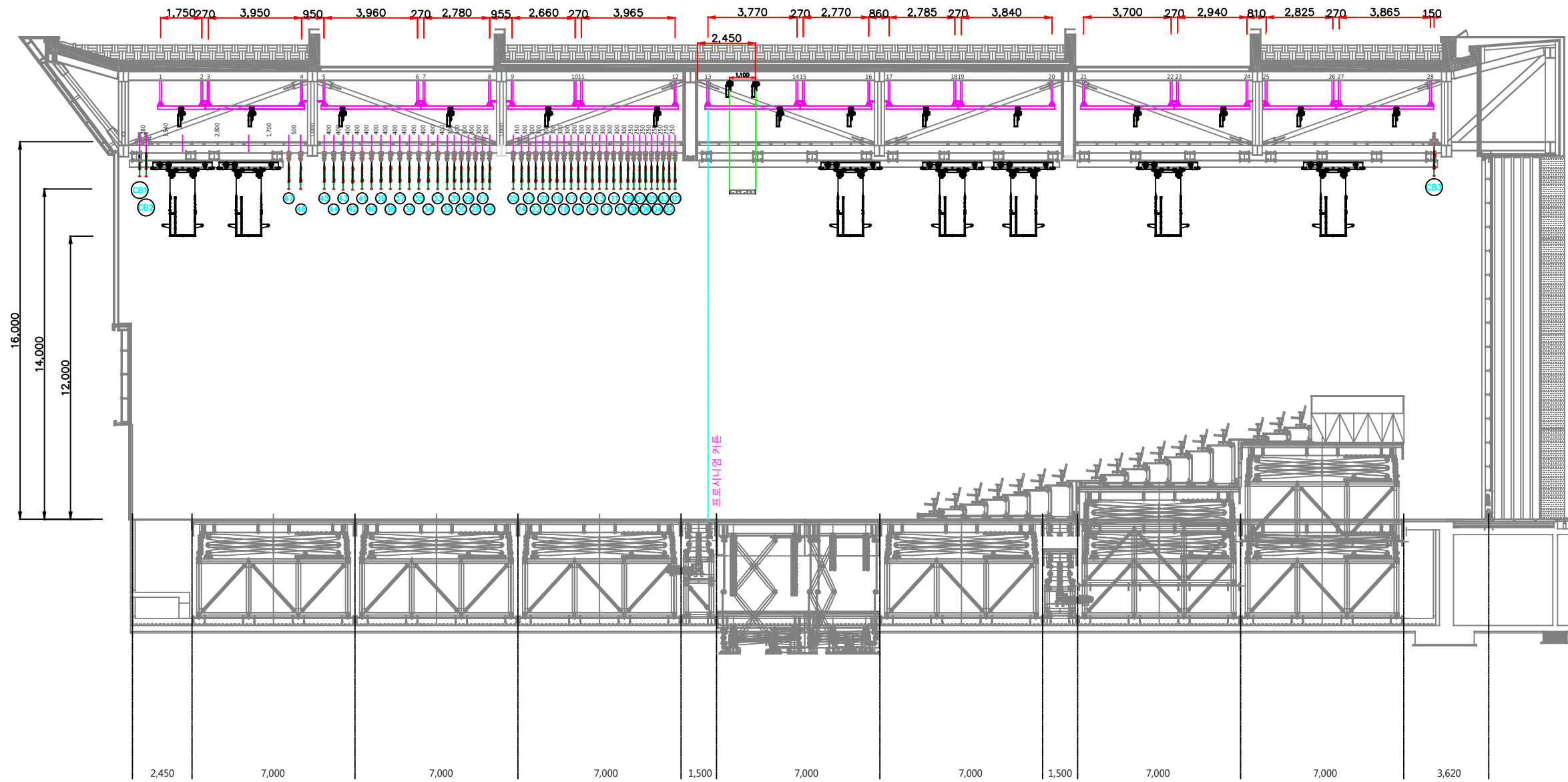
예술극장 극장1 프로시니엄 객석 측면도
